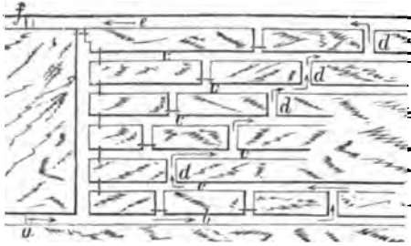
C 1771. Část větrné mapy.
